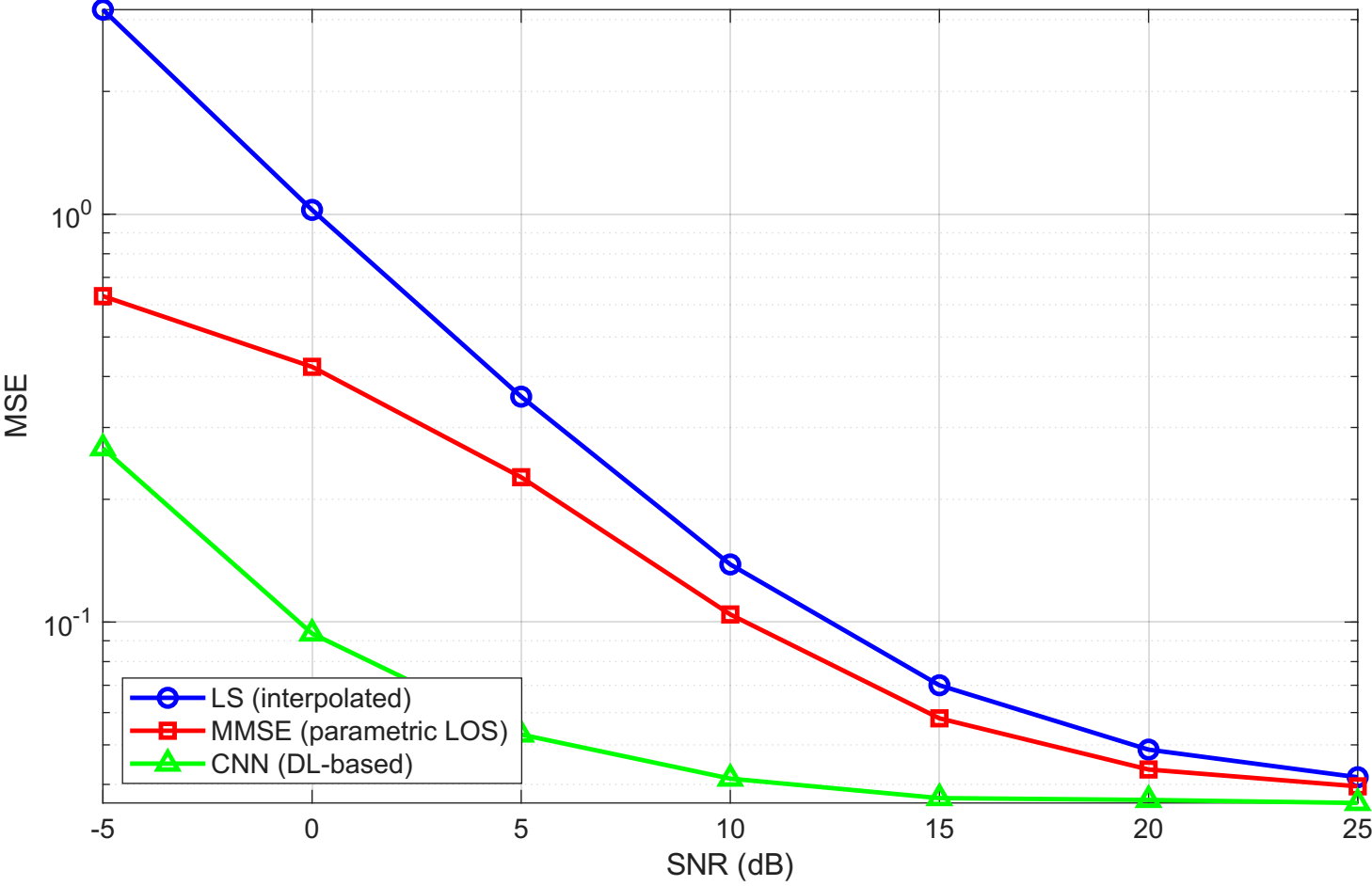
Channel Estimation MSE vs SNR — 5G NTN LOS
